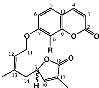
(1) R=OCH 3 (2) R=H
