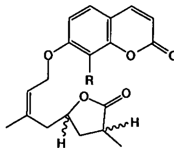
(3) R=OCH 3 (4) R=H
