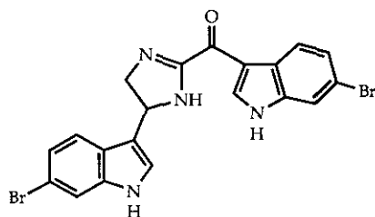
topsentine C
